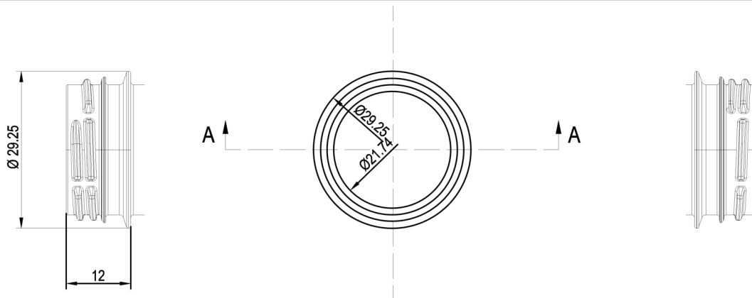
SEZIONE A-A
