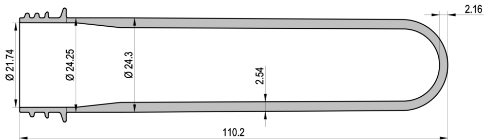
SEZIONE A-A
